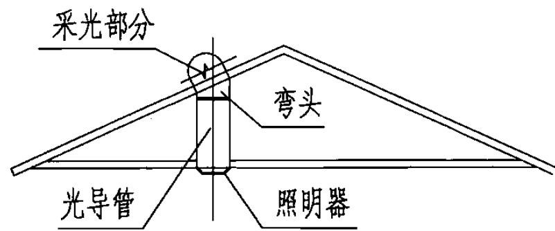
天然光导光系统的构成图
