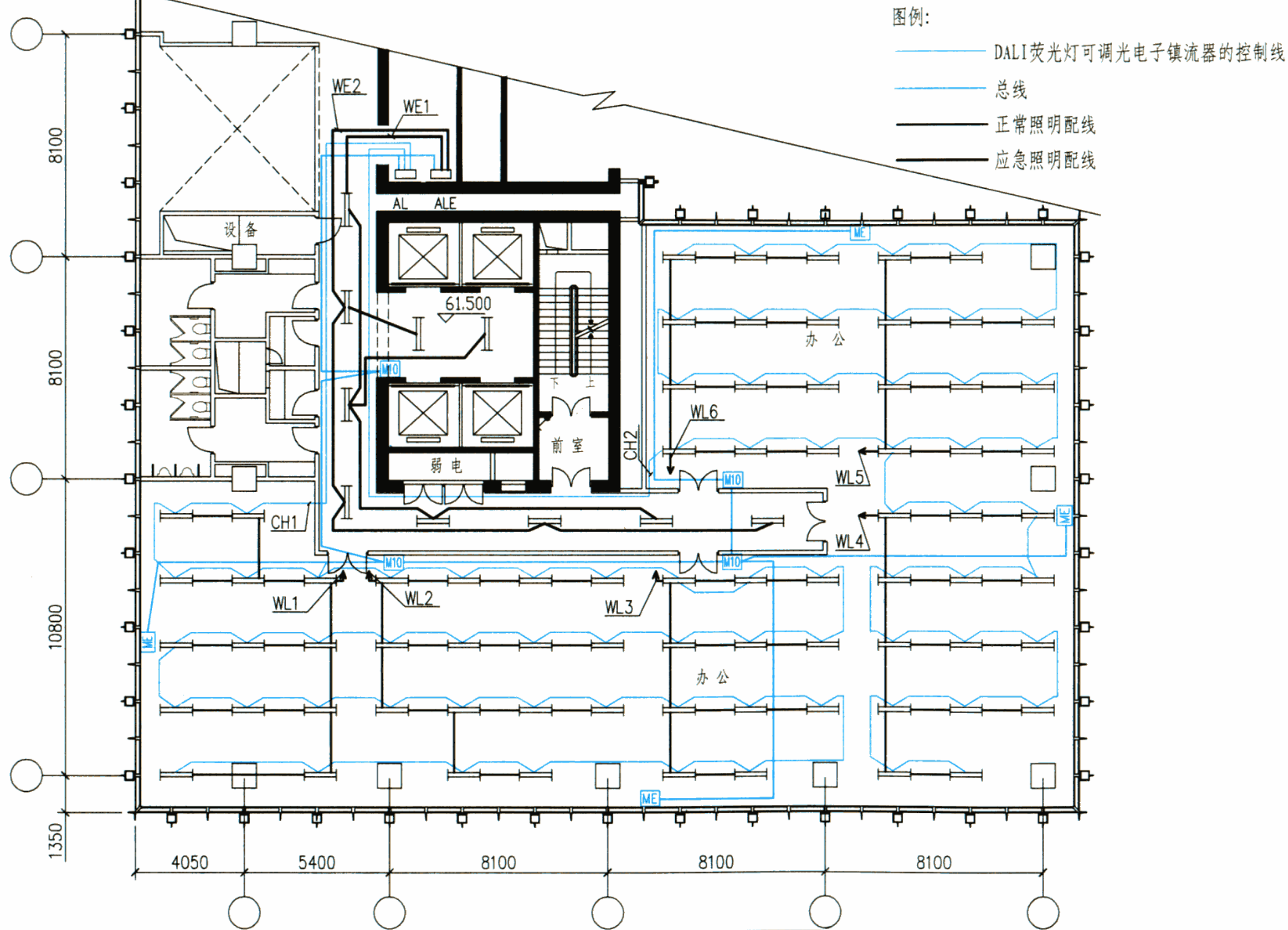
照明平面图
