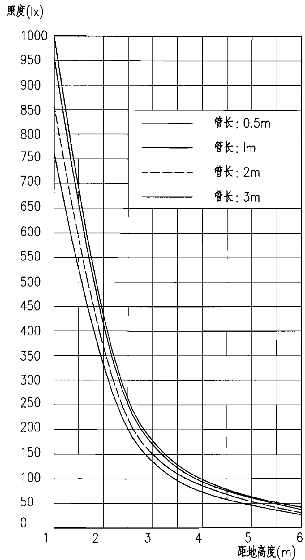
光导管距地高度与照度的关系 室外照度: 25000lx; 管径: 450mm; 反射率: 95%
