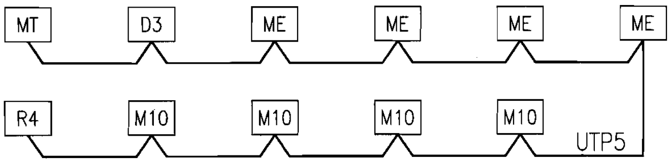
照明控制系统图
