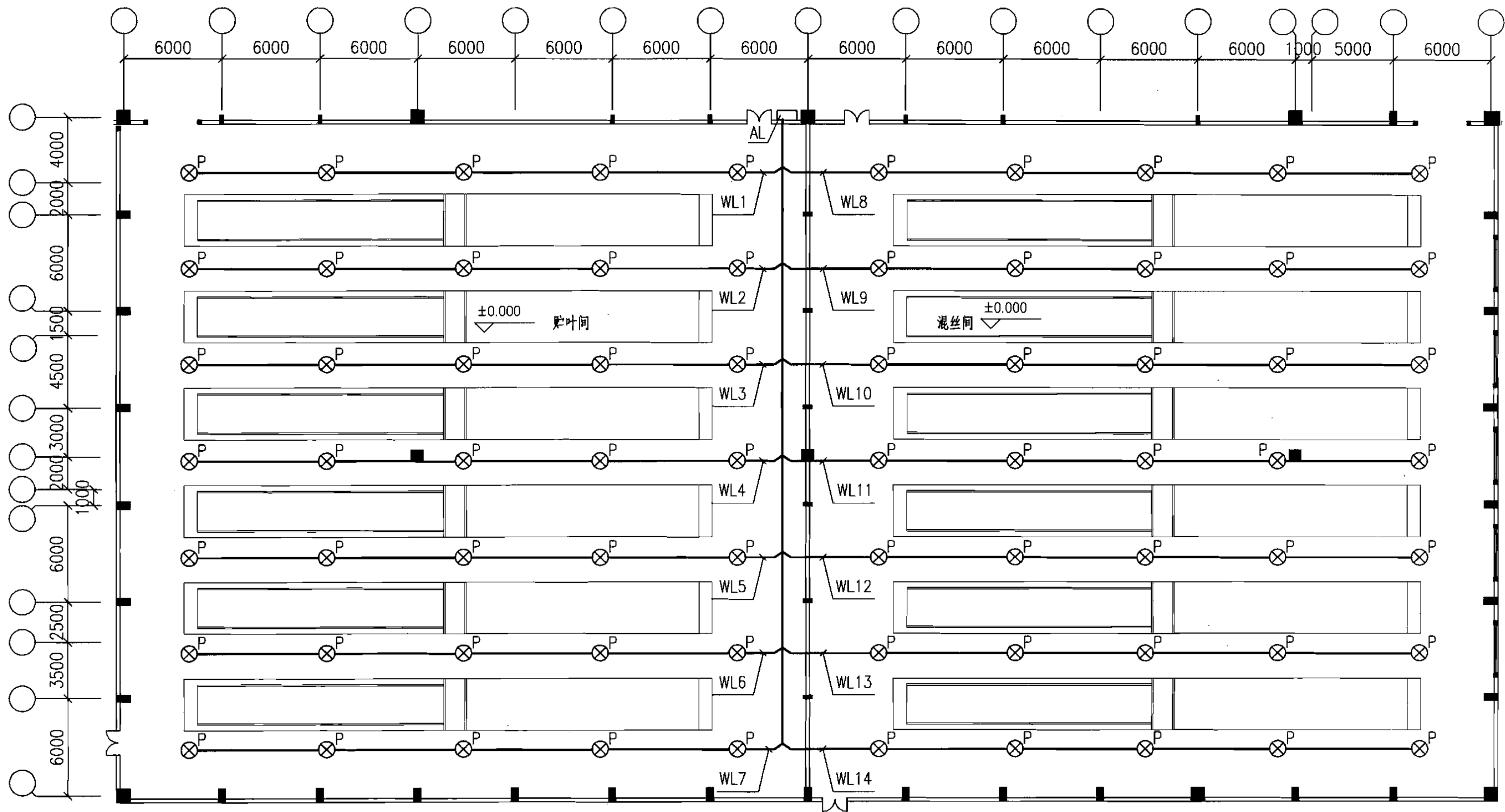
照明平面图
