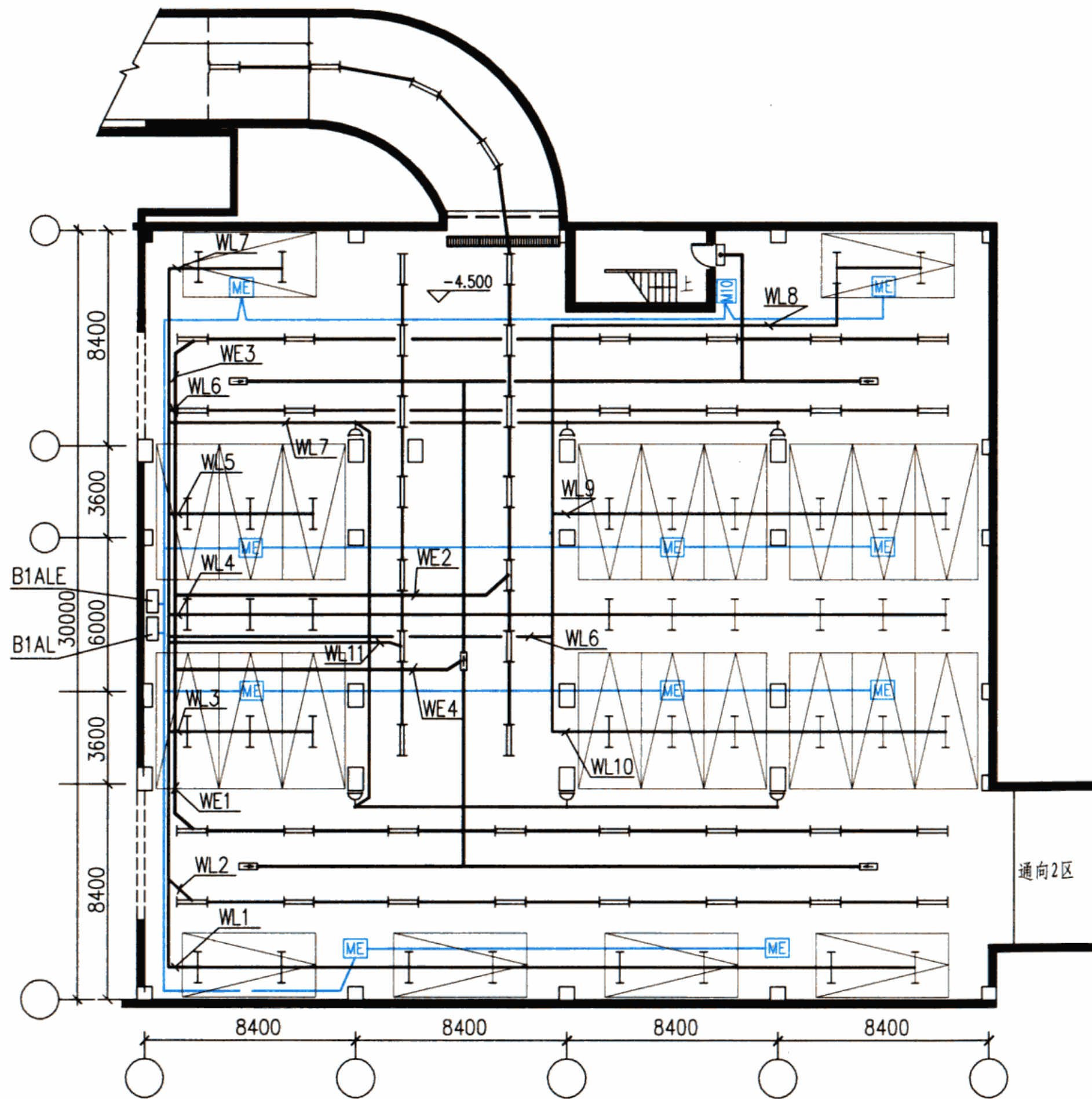
照明平面图
