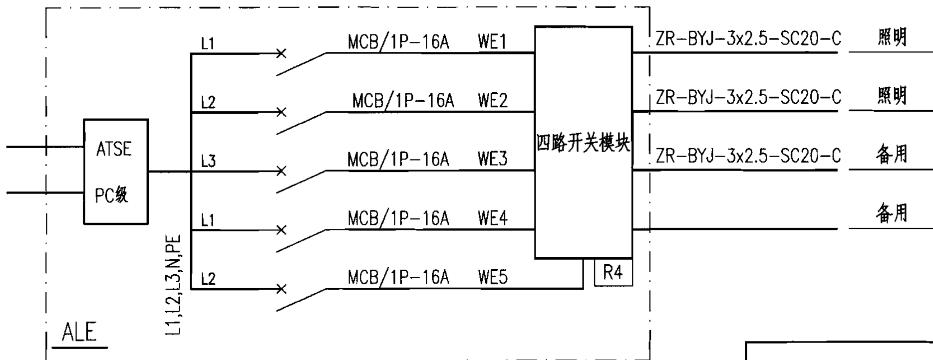
系统图
