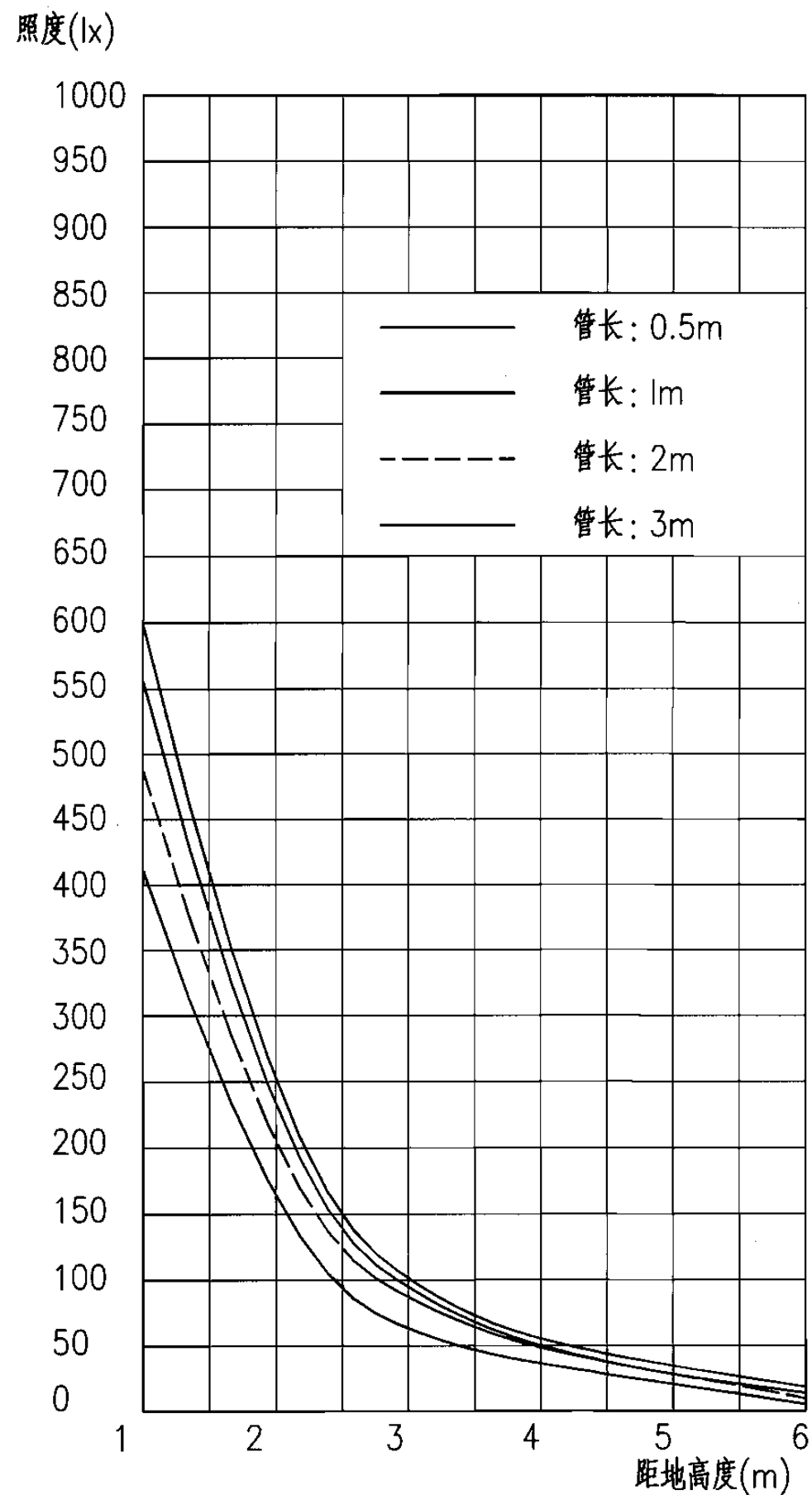
光导管距地高度与照度的关系 室外照度: 25000lx; 管径: 350mm; 反射率: 95%
