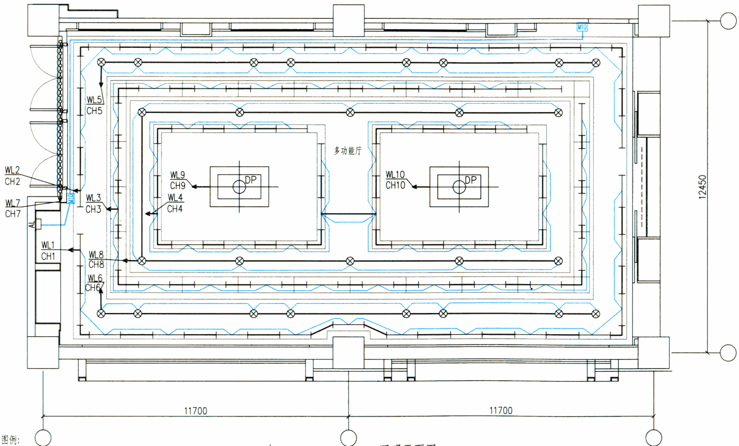
照明平面图
