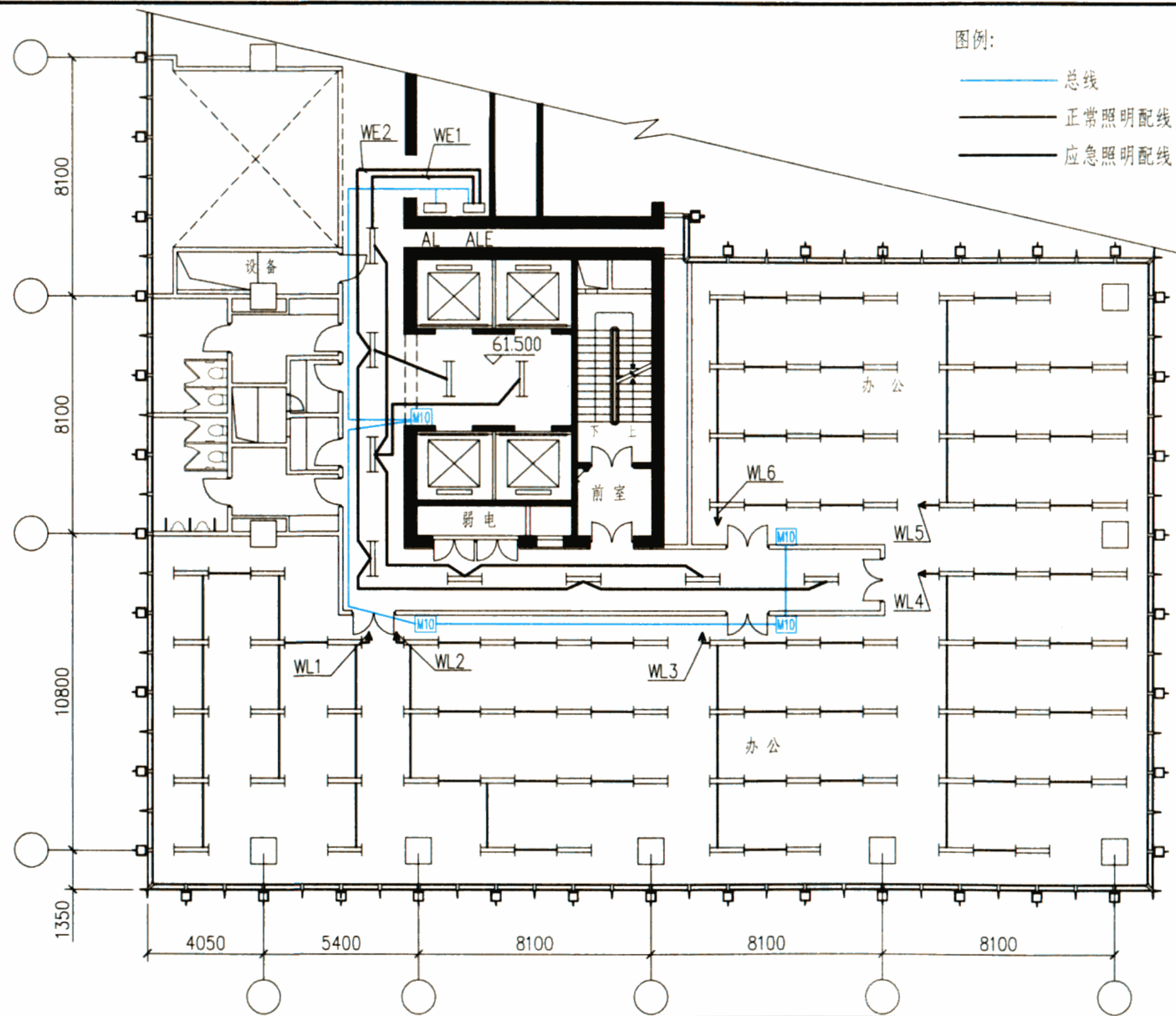
照明平面图
