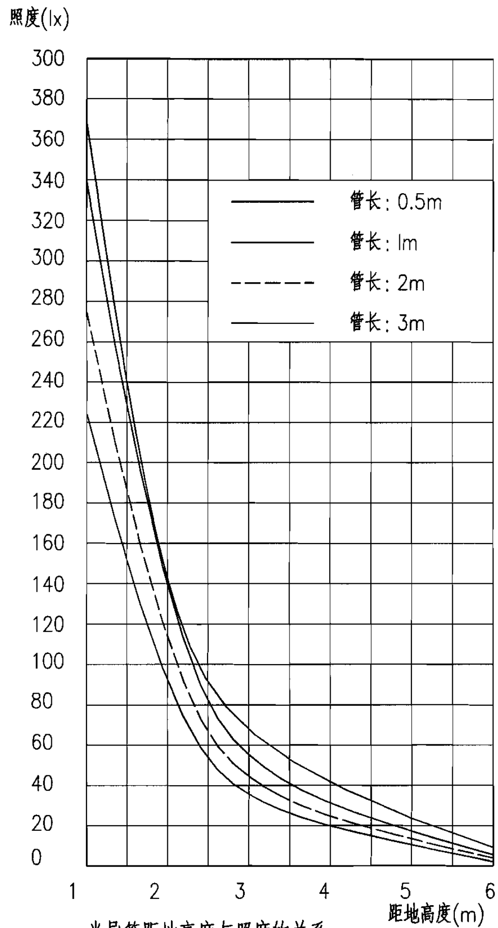
光导管距地高度与照度的关系
