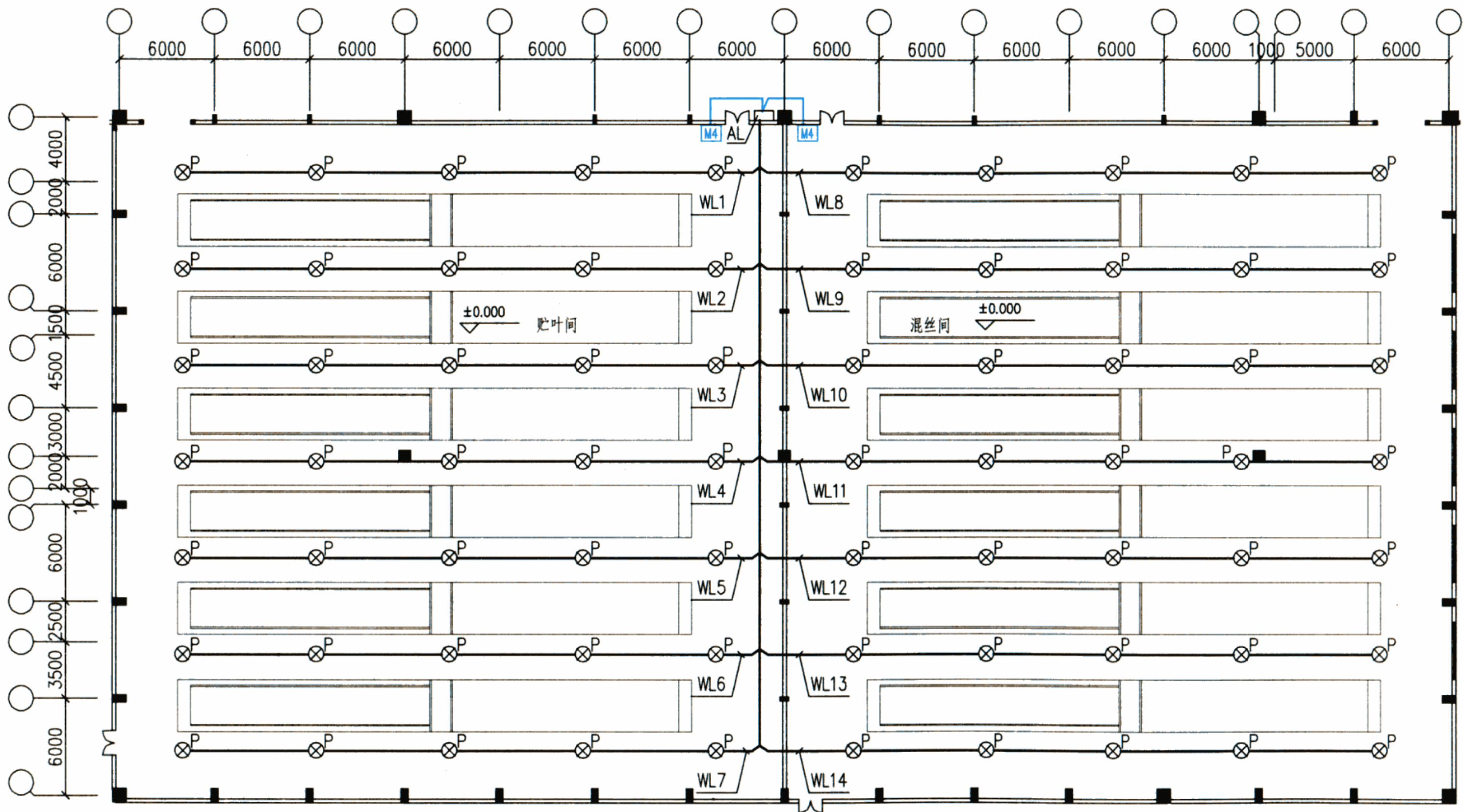
照明平面图
