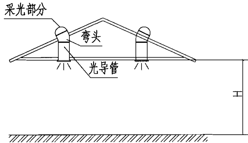
光导管布置剖面示意图
