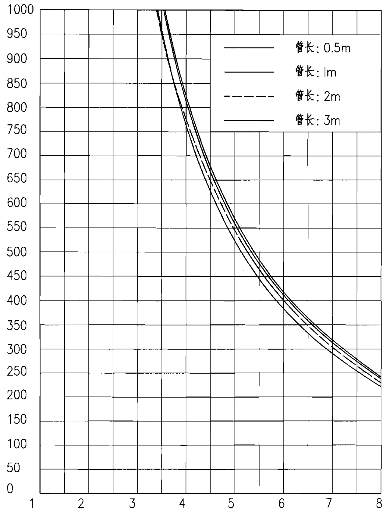
光导管距地高度与照度的关系
