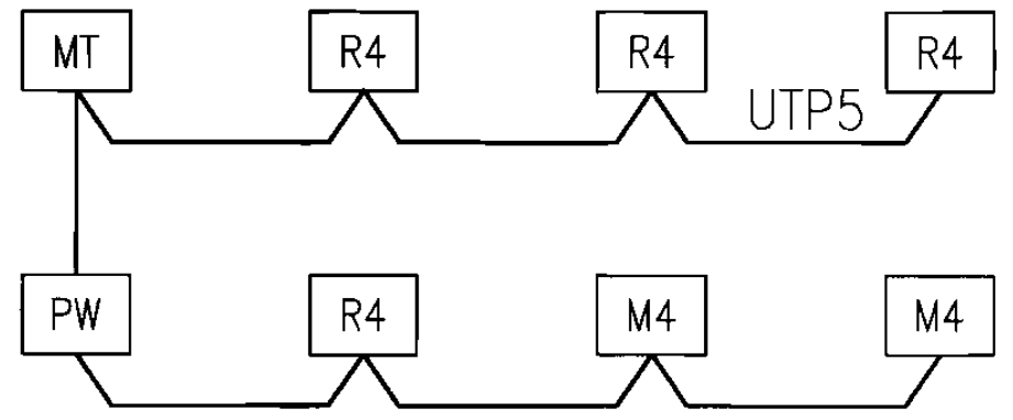
照明控制系统图
