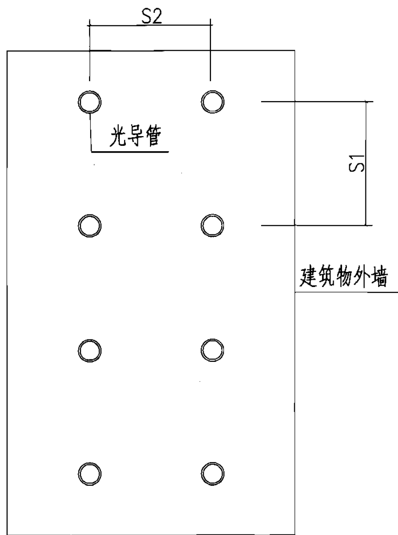
光导管布置平面示意图
