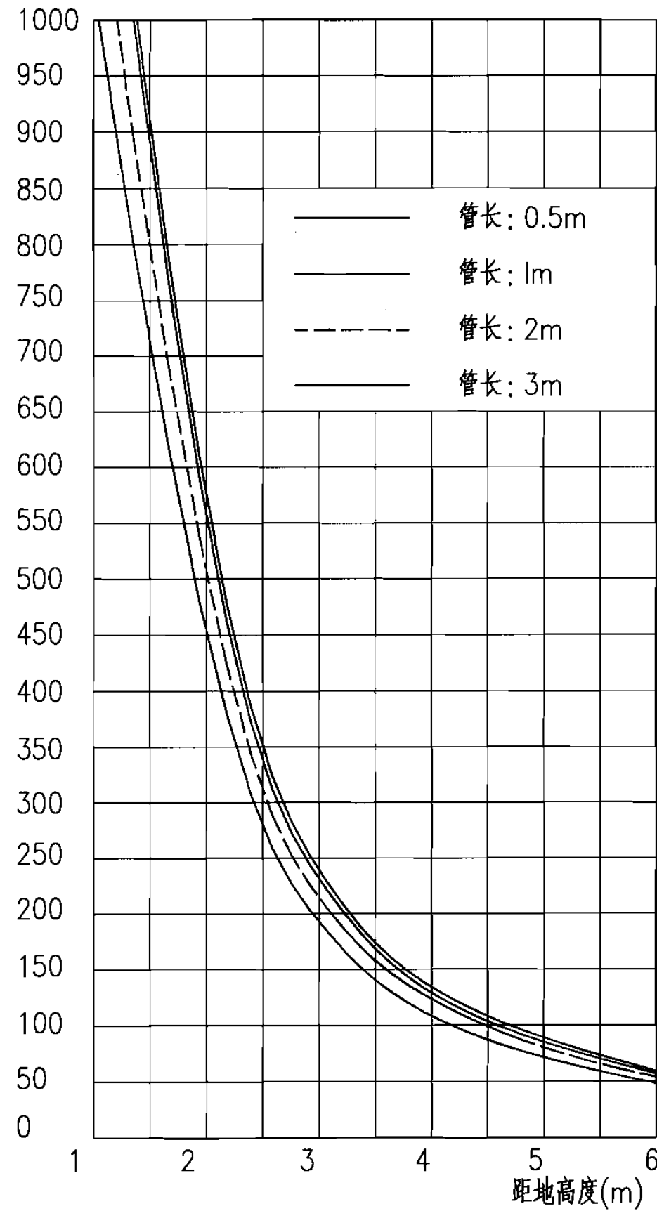
光导管距地高度与照度的关系
